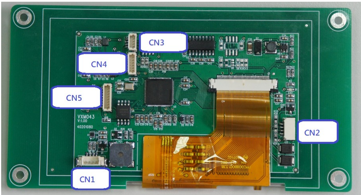
HM43-x 背面
