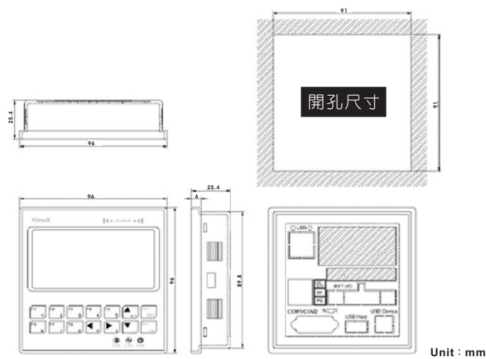
機器開孔尺寸【單位：mm】
